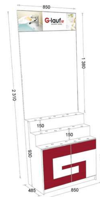
СТЕНД ДЛЯ СМЕСИТЕЛЕЙ АРТИКУЛ: ADV-1001
