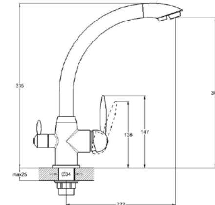
СМЕСИТЕЛЬ ДЛЯ КУХОННОЙ МОЙКИ С БИКАНАЛЬНЫМ ИЗЛИВОМ Артикул: GOR18-A093
