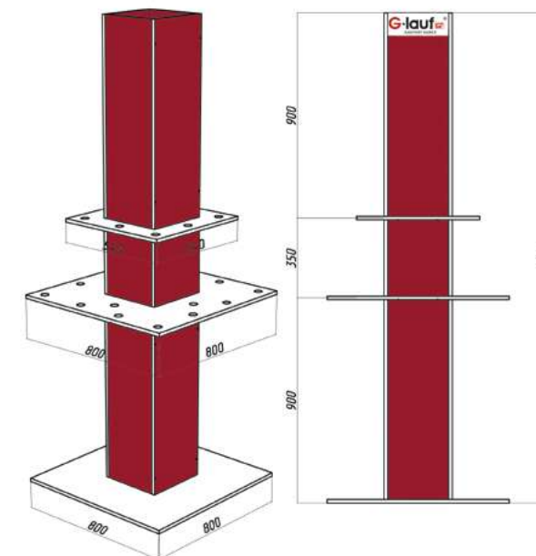
СТЕНД ДЛЯ СМЕСИТЕЛЕЙ АРТИКУЛ: ADV-1005
