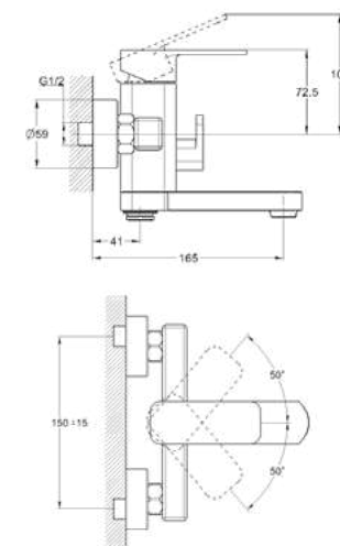
СМЕСИТЕЛЬ ДЛЯ ВАННЫ С ЛИТЫМ ПОВОРОТНЫМ ИЗЛИВОМ 125MM АРТИКУЛ: NEB3-A123 СТАРЫЙ АРТИКУЛ: LEB-3123
